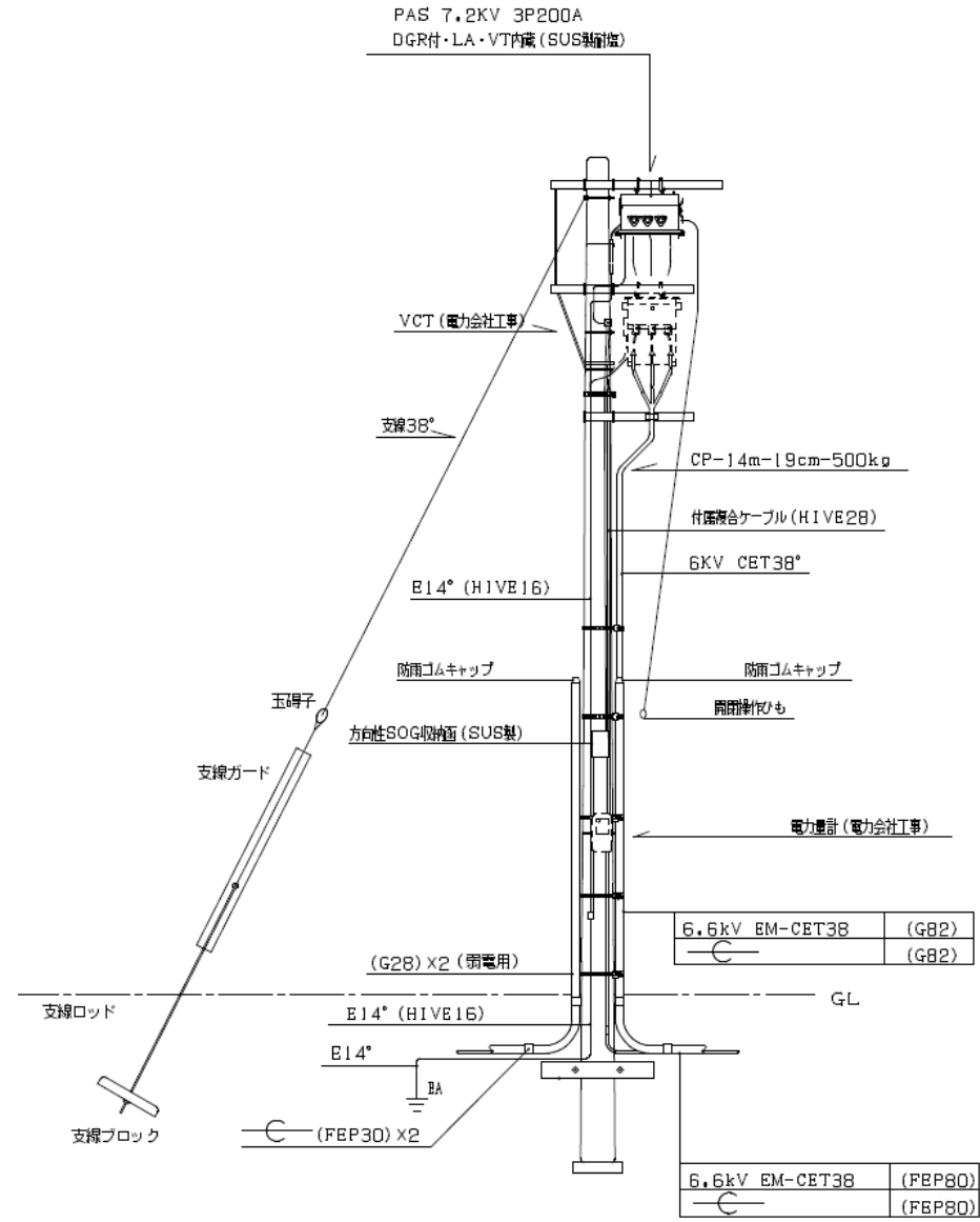
構内引込柱: 参考詳細図 (No scale)
